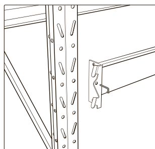
Рис 3. Установка балки на раму
