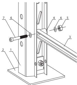
Рис 2. Установка раскосов. (1 — стойка, 2 — подпятник, 3 — горизонтальный раскос, 4 — втулка 20 мм, 5 — гайка М8, 6 — шайба М8, 7 — болт М8х55)
